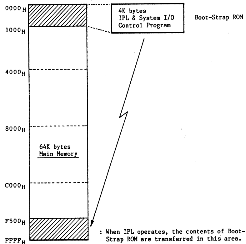
Fig. 15 : Memory Allocation
