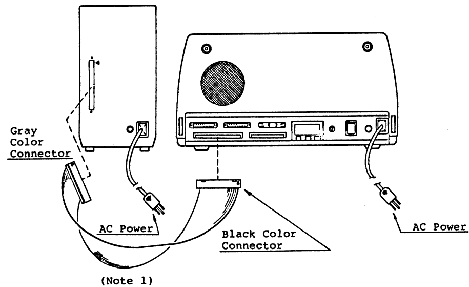
Fig. 12 : FD-8 Cable Connection
