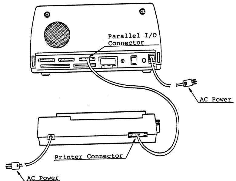
Fig. 13 : FP-80 External Printer
