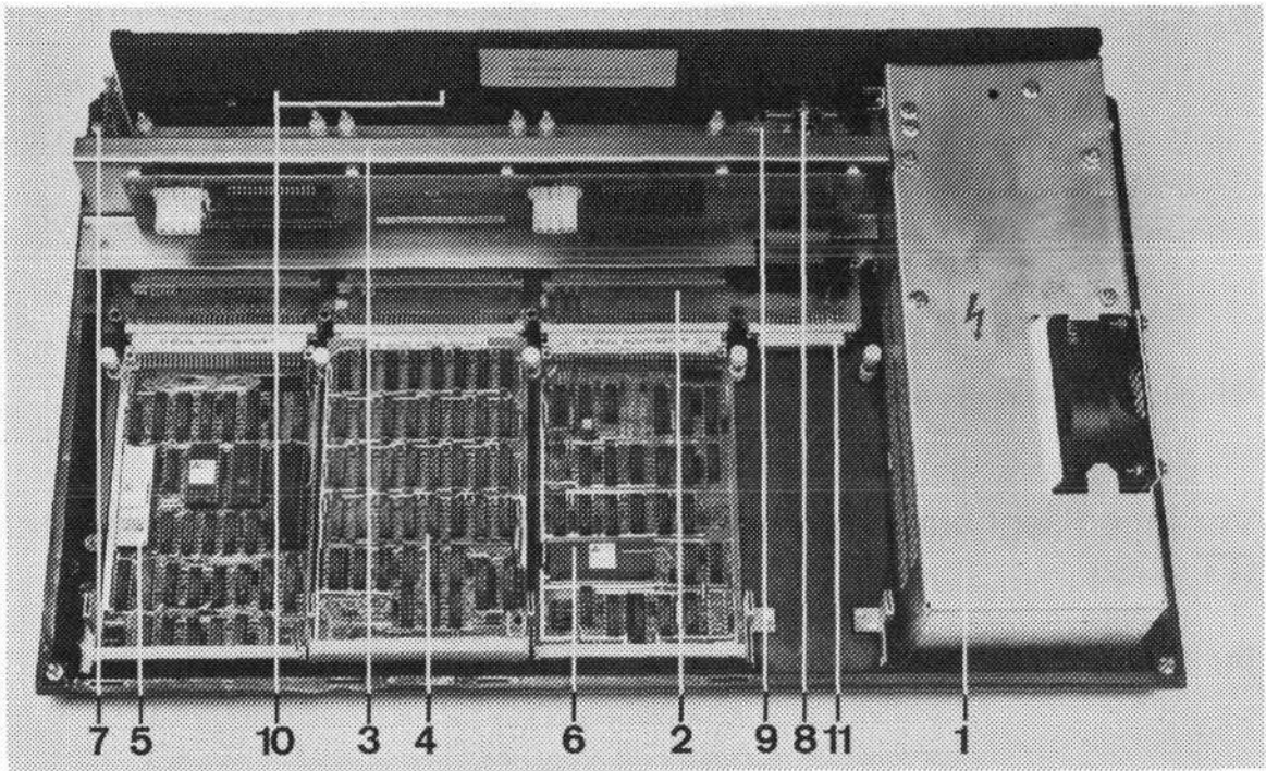
Abbildung 2: 1. Netzteil 2. Verdrahtungsfeld 3. Floppy-Halgebügel 4. CPU-Karte und Speicherkarte* 5. Video/Keyboard-Interface* 6. Floppy-Controller* 7. Tastatur-Anpassung 8. Monitor-Anschluß 9. Serielle Schnittstelle 10. Erweiterungs-Slots 11. Platz für Echtzeit-Ihr*, Arithmetik-Baustein* (*ist je nach Lieferumfang zu bestücken).
