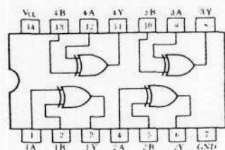
74LS86
