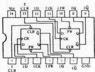
SN 74LS75
