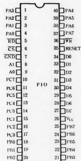
#PD8255
